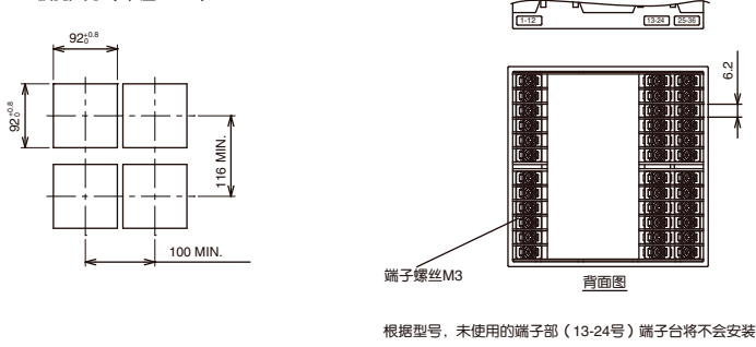
面板孔尺寸（单位：mm）
